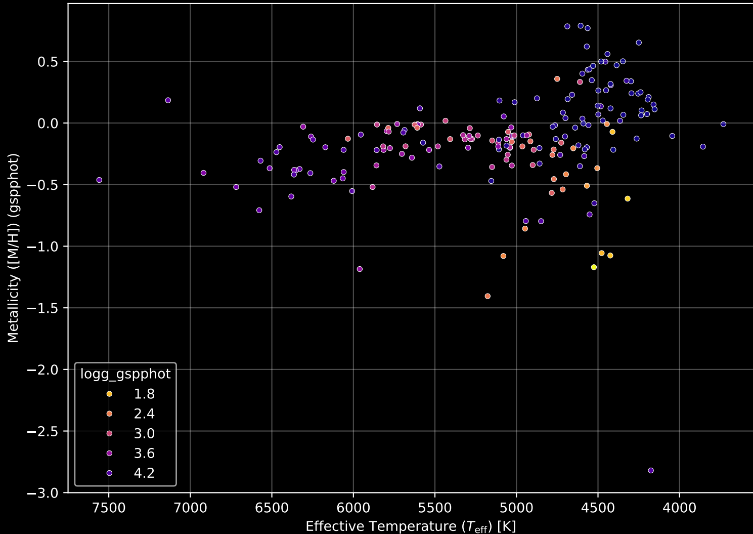
APOGEE DR17 Field: [277+76] Stellar Population Parameters (n= 184)
